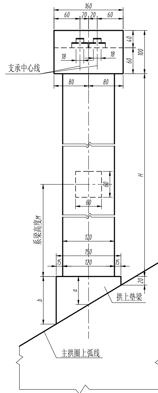
侧面图 1:50
