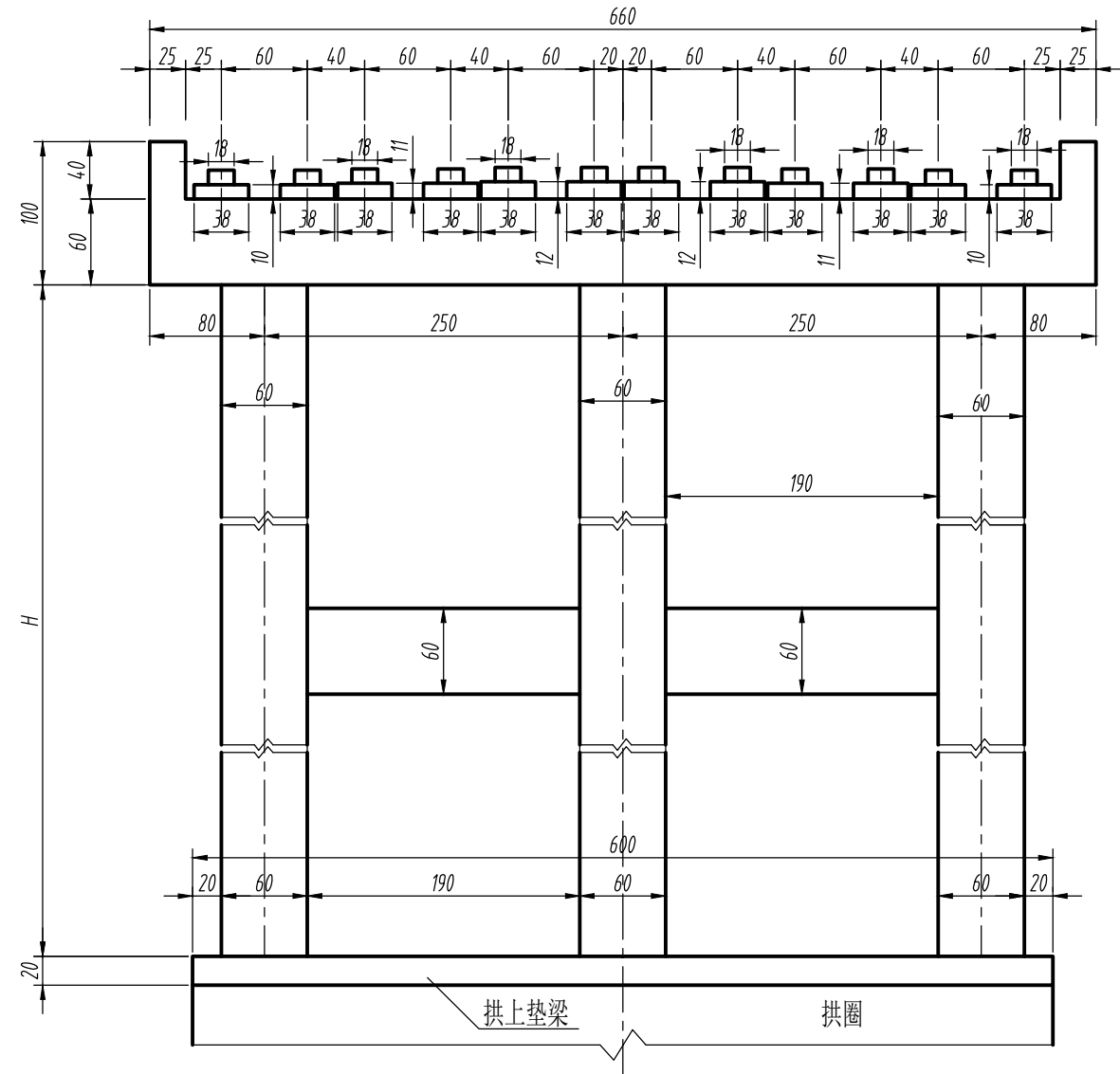
拱桥立柱及盖梁立面图 1:50
