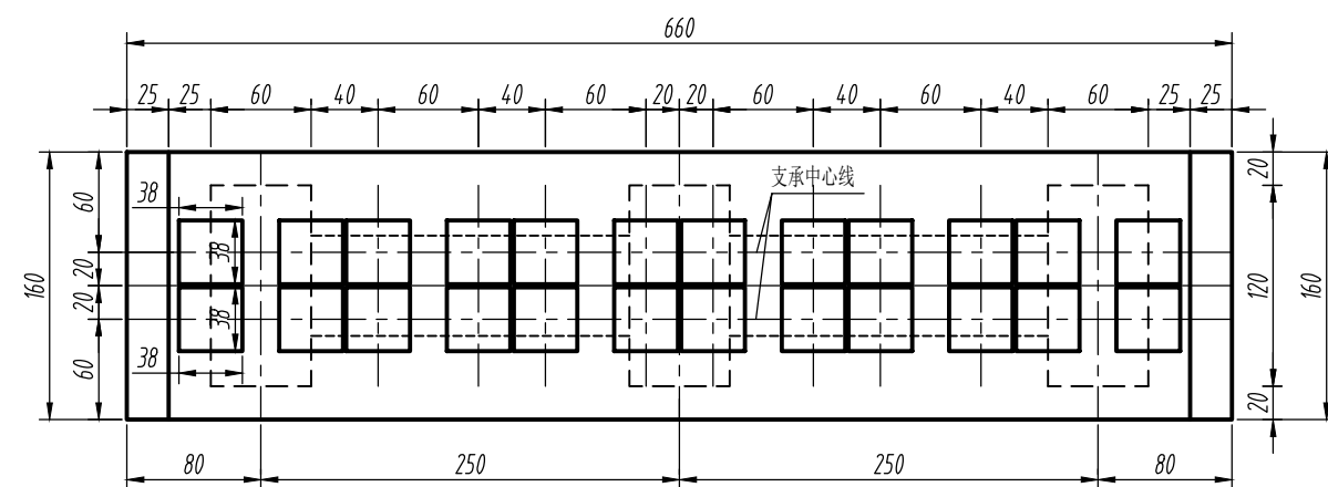
平面图 1:50
